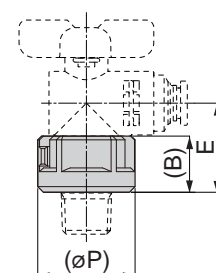
製品取付け時(正面)
