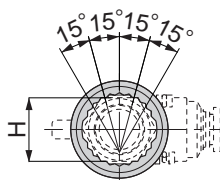
製品取付け時(下面)
